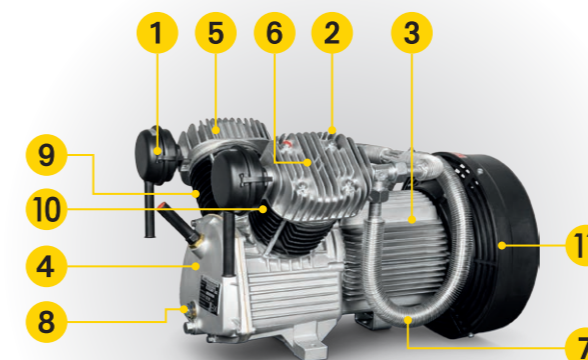
MEK
